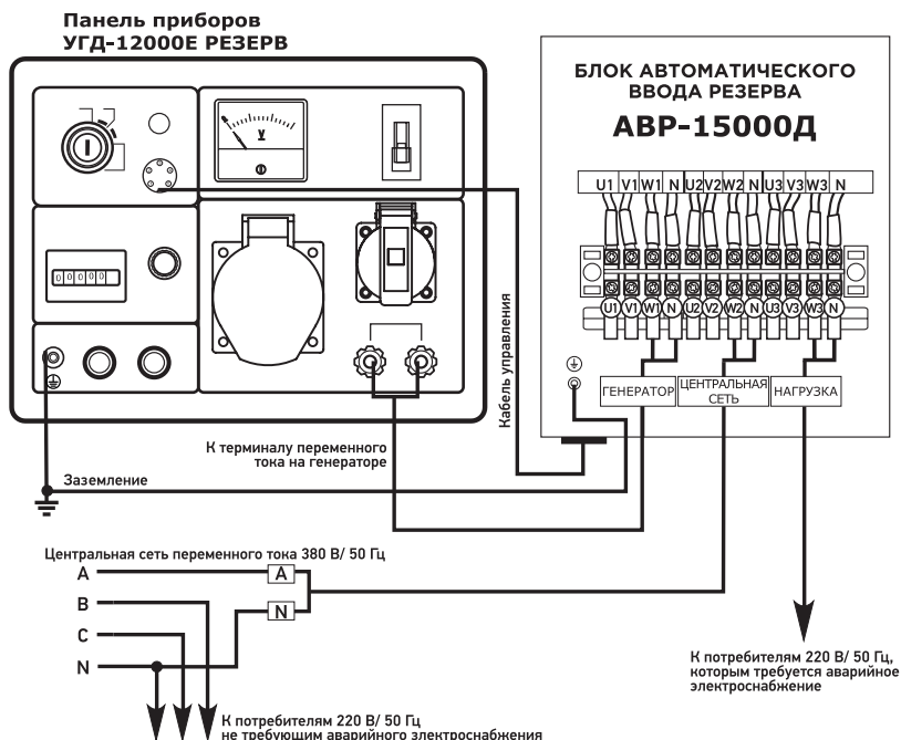
Рис. 15. Схема подключения блока АВР-15000Д и однофазного генератора на 220 В к трехфазной сети
