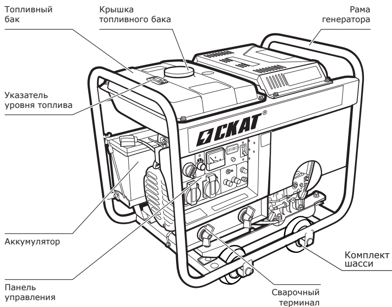
Рис. 5. Общий вид генератора УГСД-4000/180E PROFF.
