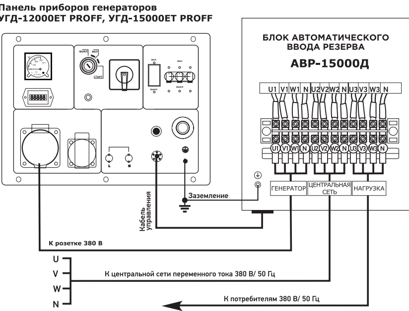
Рис. 19. Схема подключения блока АВР-15000Д к трехфазному генератору 380 В.
