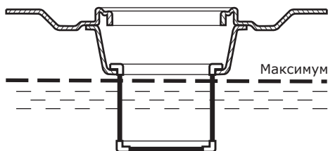
Рис. 11. Заполнение топливного бака и контроль уровня топлива.
