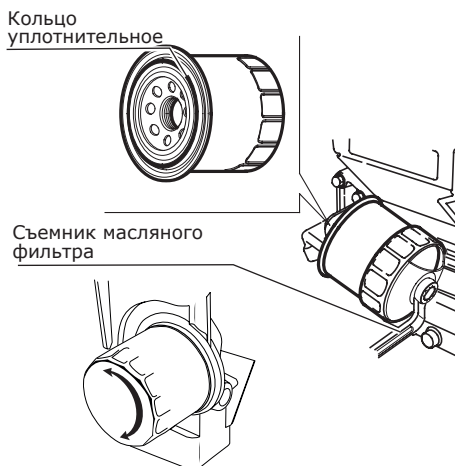
Рис. 24. Замена масляного фильтра.
