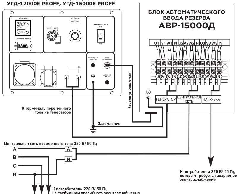
Рис. 20. Схема подключения блока АВР-15000Д и однофазного генератора на 220 В к трехфазной сети.
