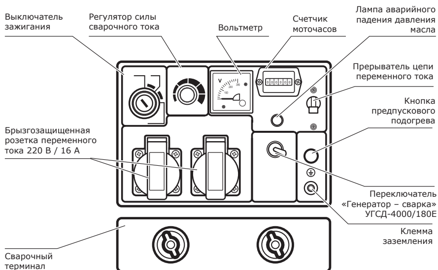
Рис. 6. Схема панели управления генератора УГСД-4000/180E PROFF.
