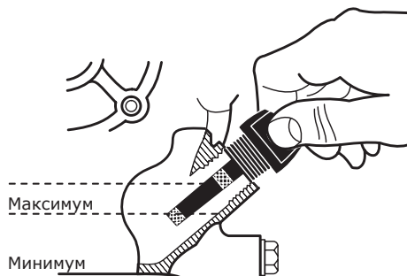
Рис. 7. Заполнение масляного картера и контроль уровня масла.
