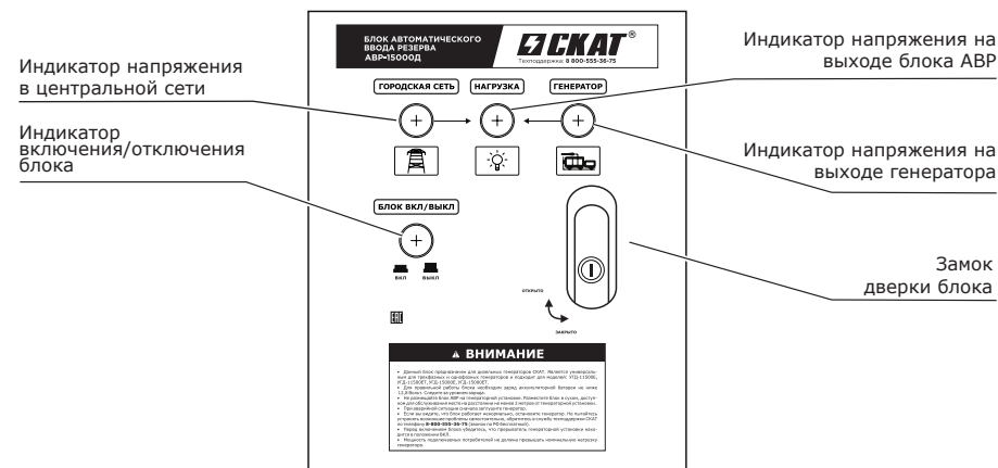
Рис. 17. Внешний вид и схема панели управления блока автоматического ввода резерва
