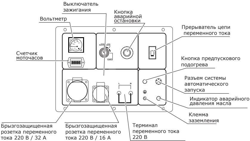
Схема панели управления генераторов УГД-11500Е PROFF, УГД-15000Е PROFF.
