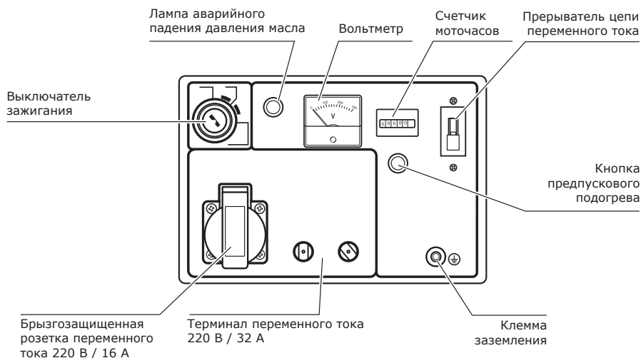
Схема панели управления генераторов УГД-9500Е PROFF, УГД-11000Е PROFF.
